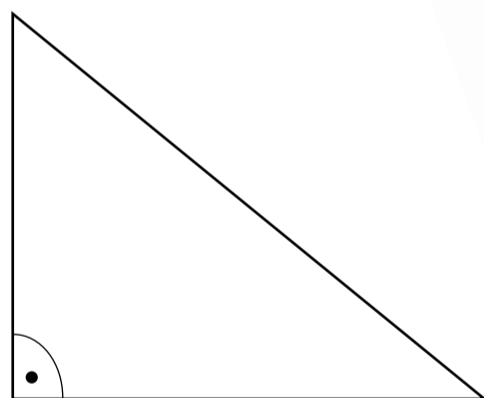
Правоъгълен
