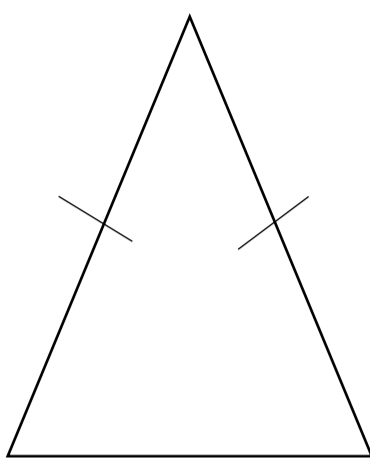
Равнобедрен
