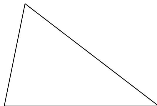
Разностранен
