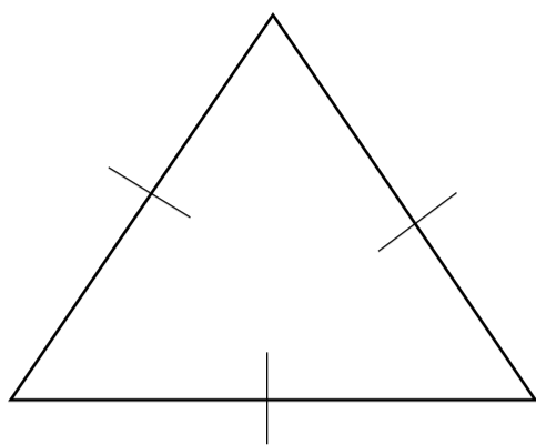
Равностранен
