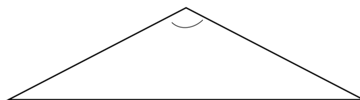
Тъпоъгълен
