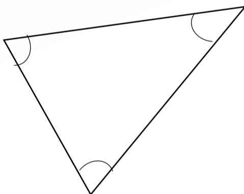
Остроъгълен
